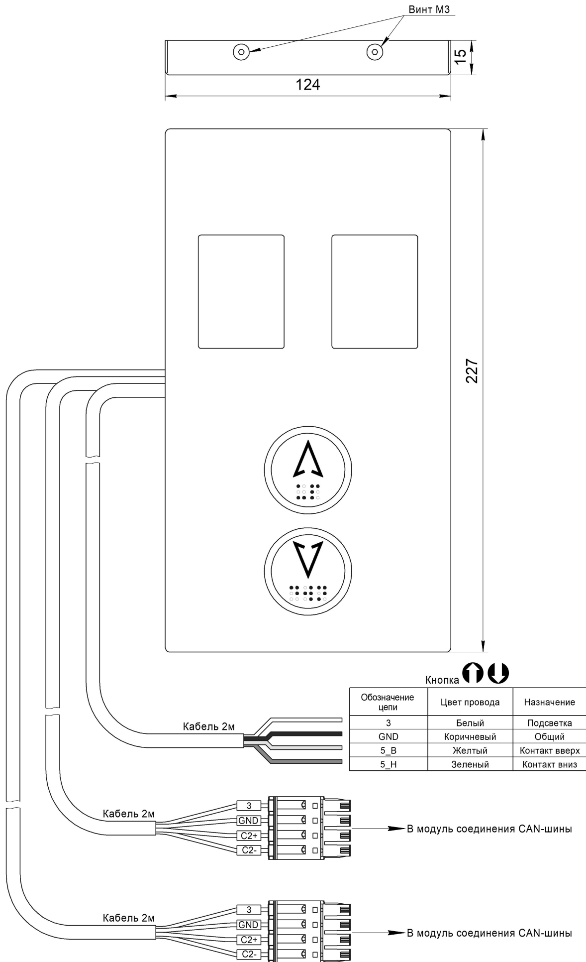
Рис.1 Внешний вид, габаритные и установочные размеры Вызывного поста ВП-2103-2086-10
